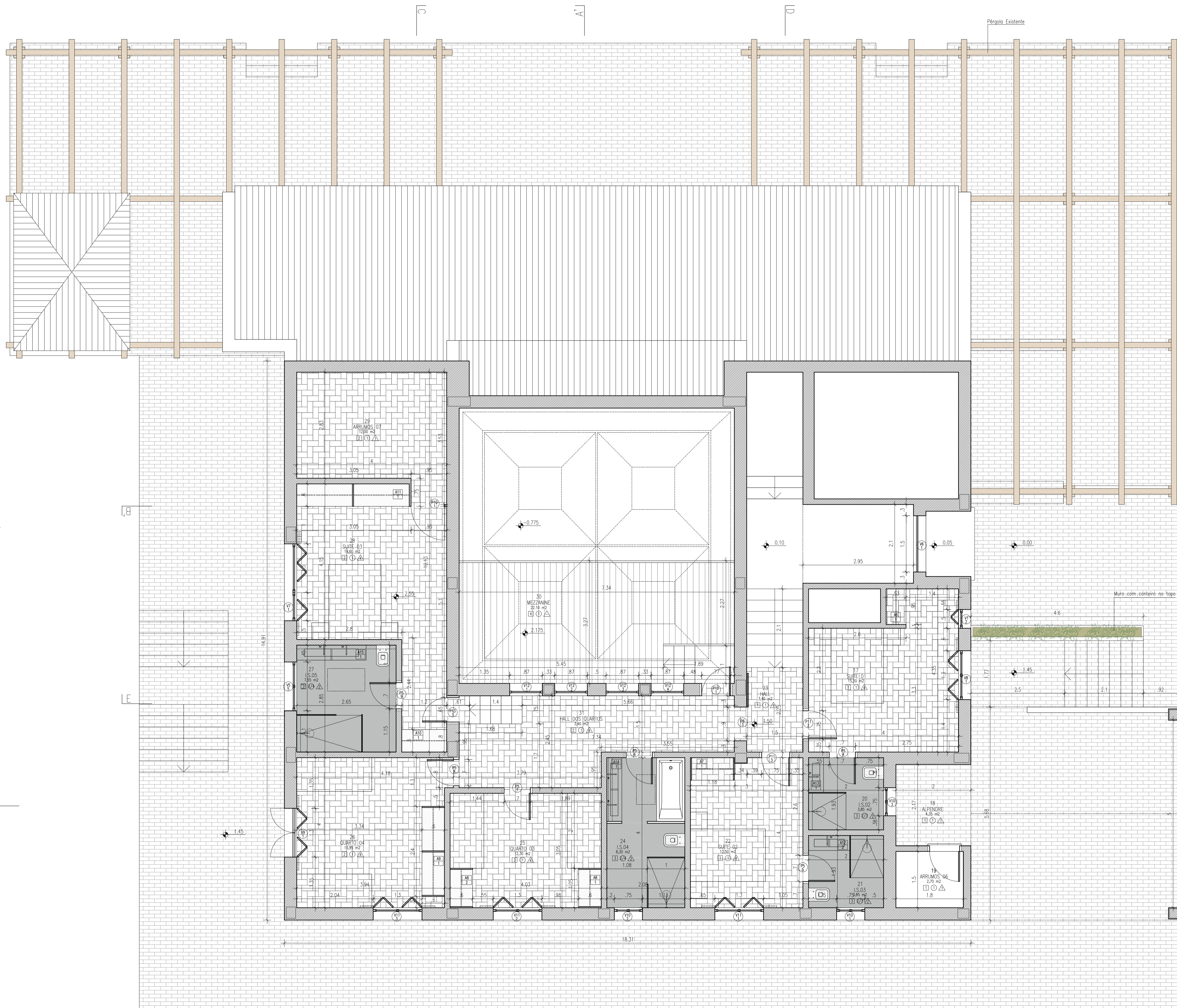
PLANTA PISO 1 (COTA 3.60M)
